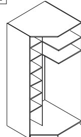
Ormar kutni RKKT 98,6-96,6-232,4
