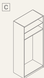
Ormar široki, 2 stranice TKO100H 102,7-60-232,4
